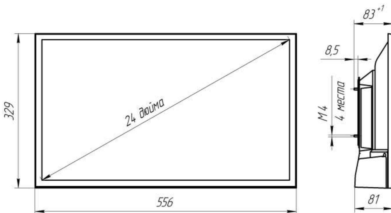
Рисунок 1 – Общий вид и габаритные размеры телевизора.
