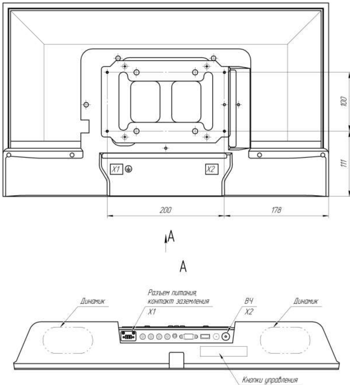
Рисунок 2 – Вид сзади. Присоединительные размеры.
