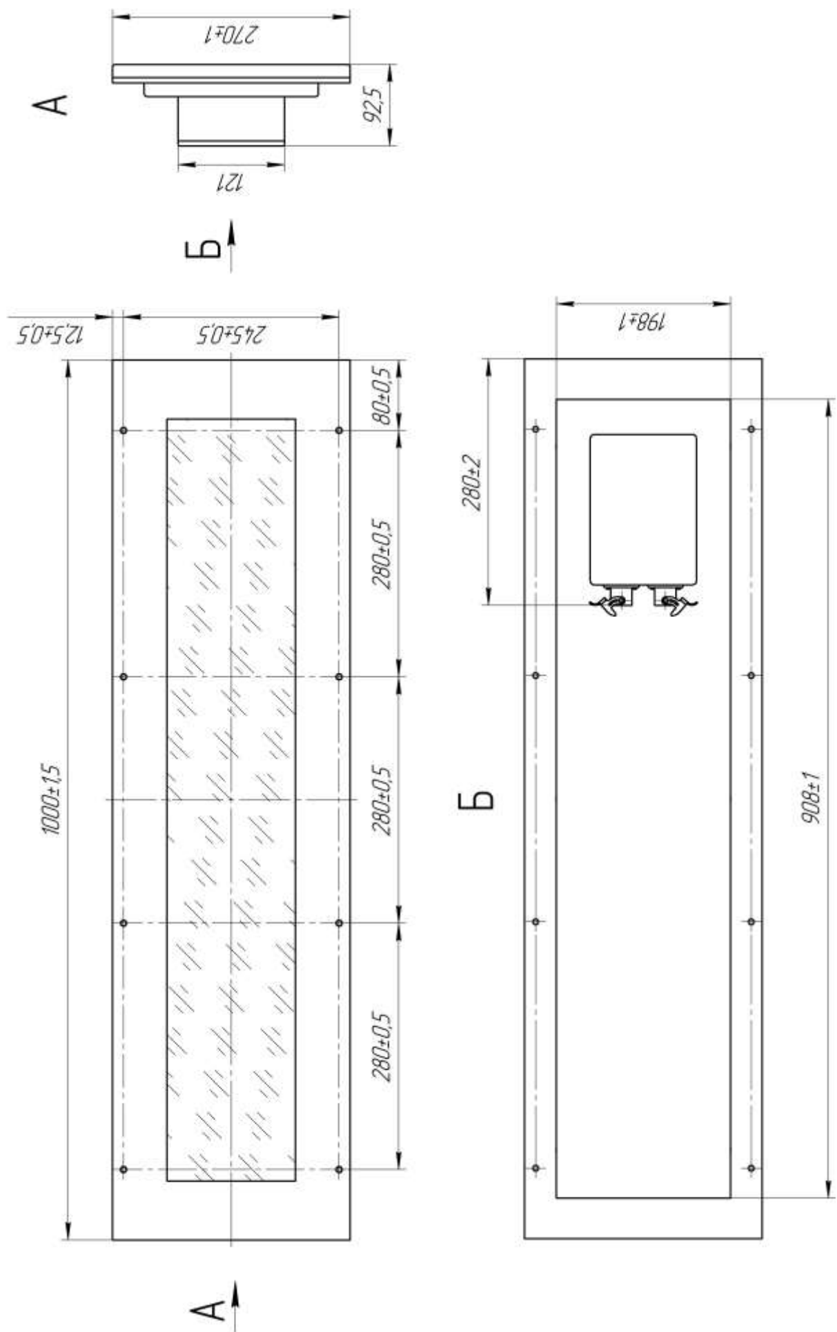
Рисунок 1 - Габаритные размеры панели маршрутной ПМЛ-110-06
