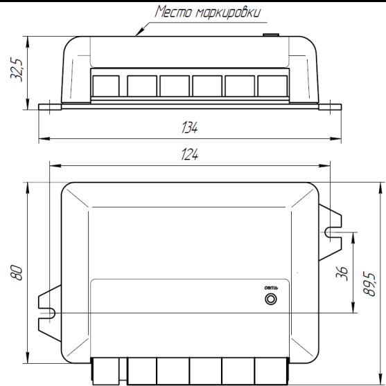
Рис.2 Габаритные и присоединительные размеры AP-1x4
