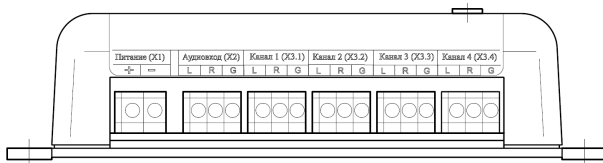
Рис.1 Маркировка разъемов AP-1x4
