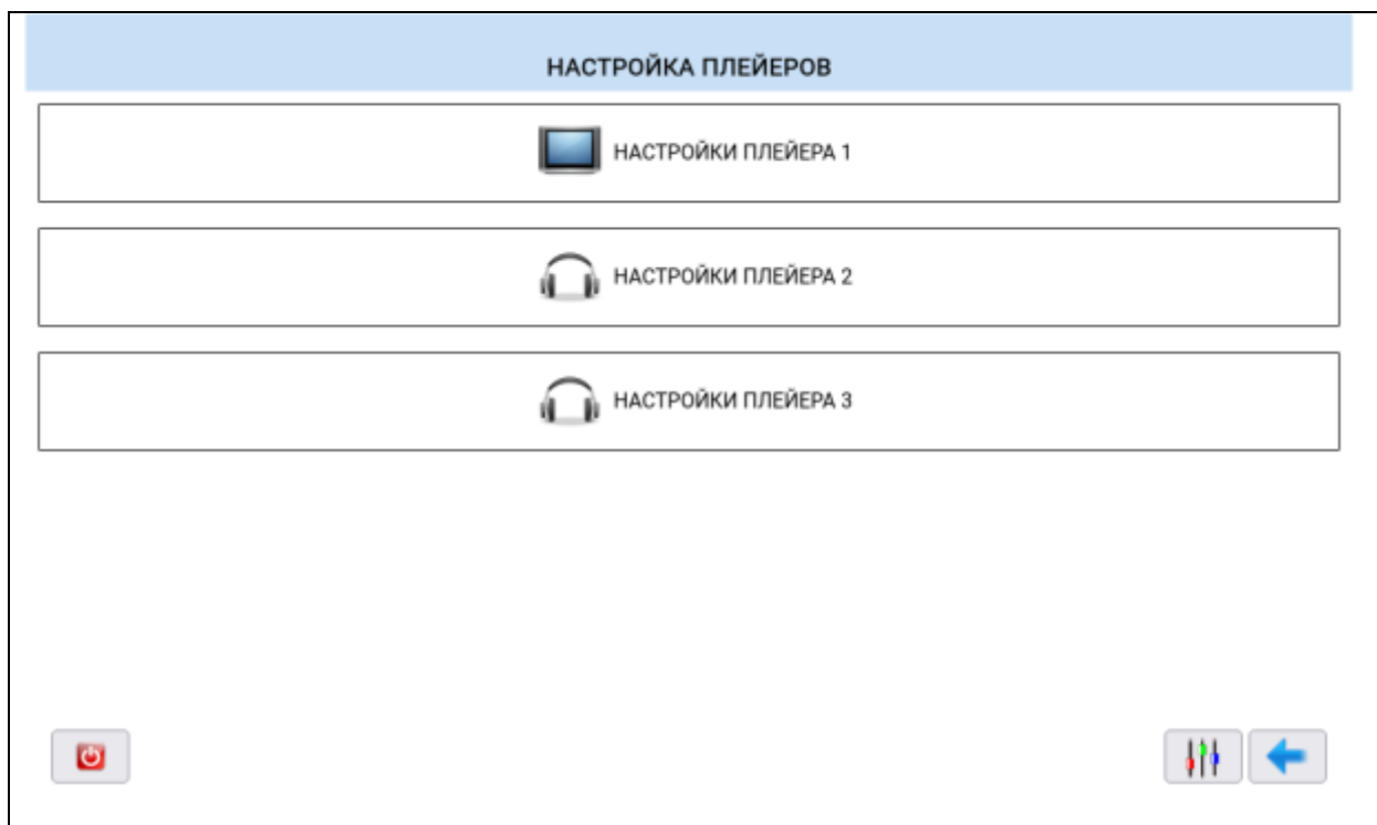
Рисунок 5 - Настройка плееров.
