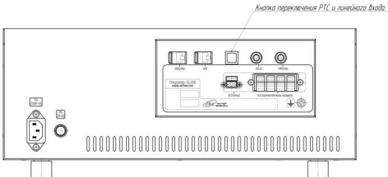
Рисунок 2 - Панель разъемов сервера-2.02.
