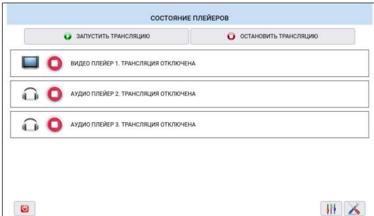
Рисунок 3 - Главное окно
