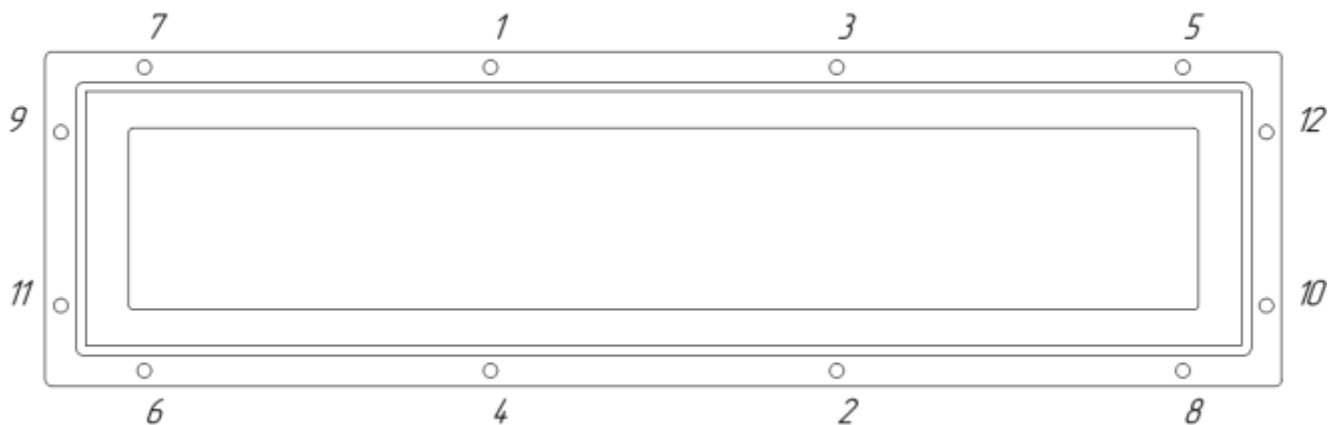
Рис. 3 – Рекомендуемая схема последовательности затяжки винтов.
